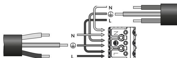
Cableado pasante
